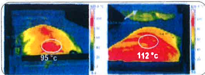
左はPVCシート、右はシリコン塗布合材シートの場合の温度
